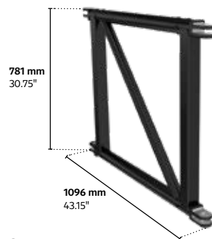
S-BTQT1018
