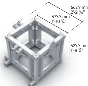
MT2-03|FTP|RTO|SleeveBlock
