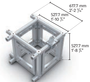
MT2-03|QTP|RTO|SleeveBlock
