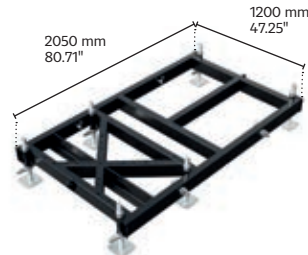
MT-IconBase-01|STEEL
